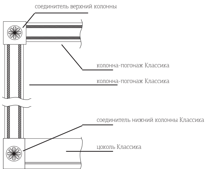
Схема установки погонажного декора Классика
