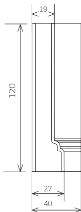
Соединитель цоколя внутренний
