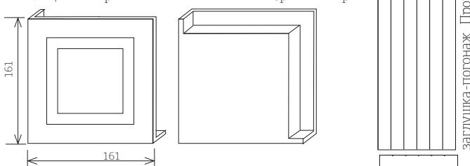
Соединитель верхний заглушки
