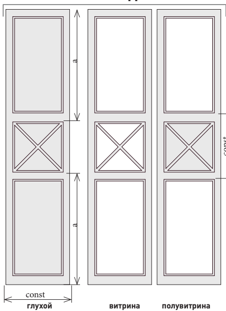
Размеры дверей Вид 3
