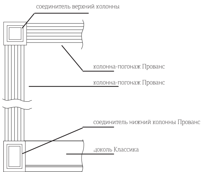
Схема установки погонажного декора Прованс
