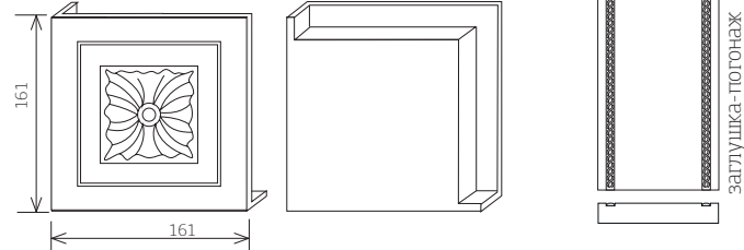
Соединитель верхний заглушки
