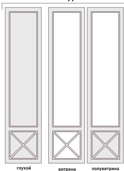
Размеры дверей Вид 2
