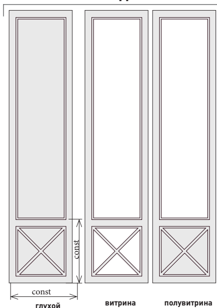
Размеры дверей Вид 2
