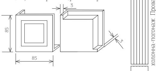
Соединитель верхний колонны
