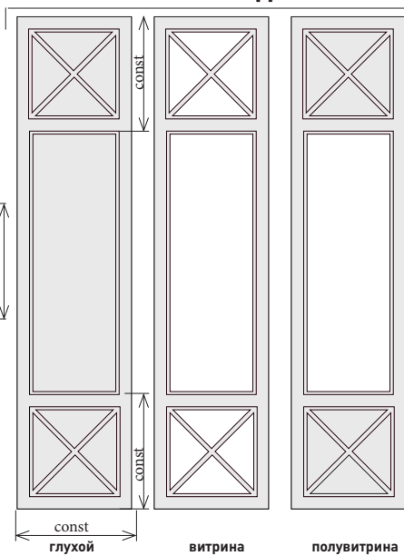
Размеры дверей Вид 4
