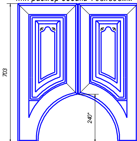
Двойка 0, 1-Элегия 703x596 мм min размер двойки 703x596мм
