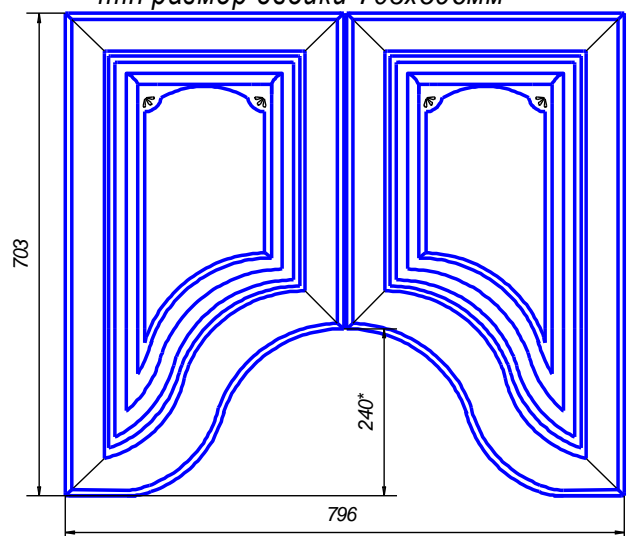
Двойка-В 0, 1-Элегия 703x796 мм min размер двойки 703x596мм
